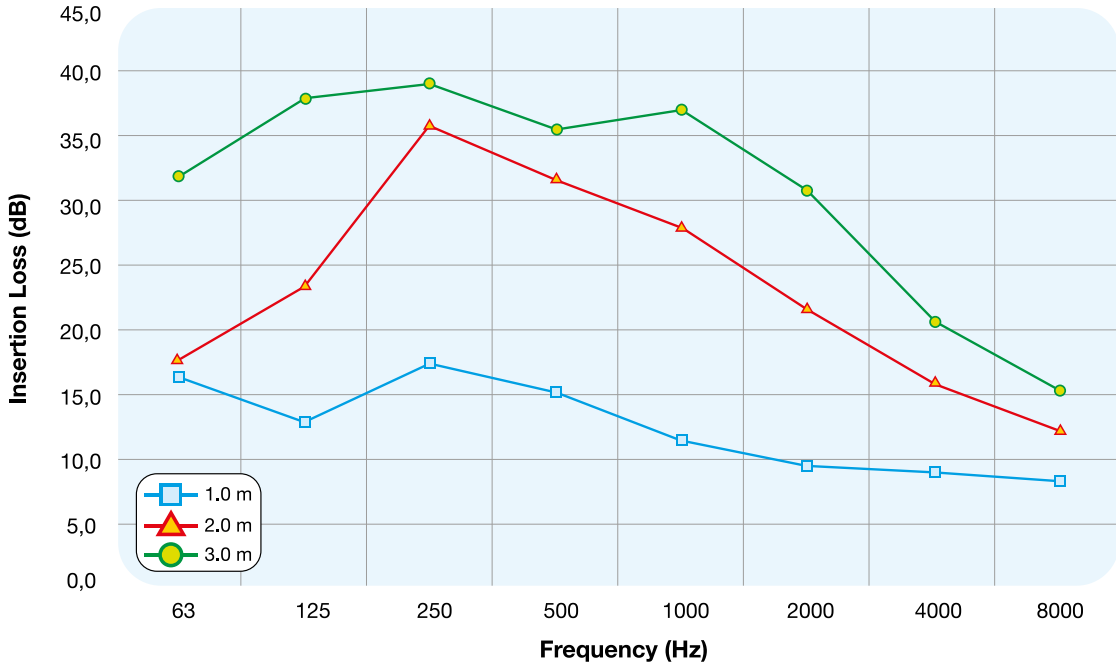
SONOAFS-ALU.F - Ø 160 mm
