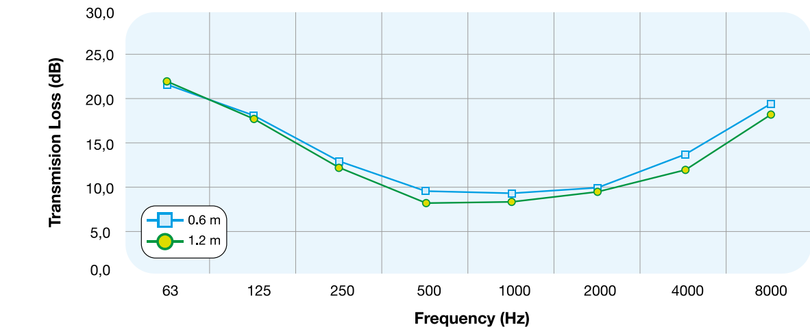
SOUNDROPAFS.P - Ø 125 mm
