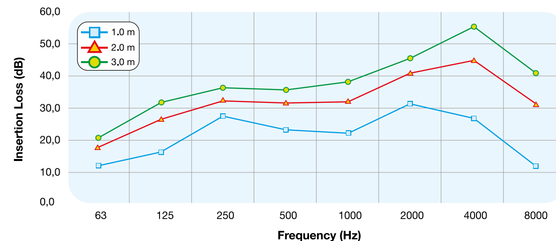
SONOAFS-NW.P - Ø 160 mm
