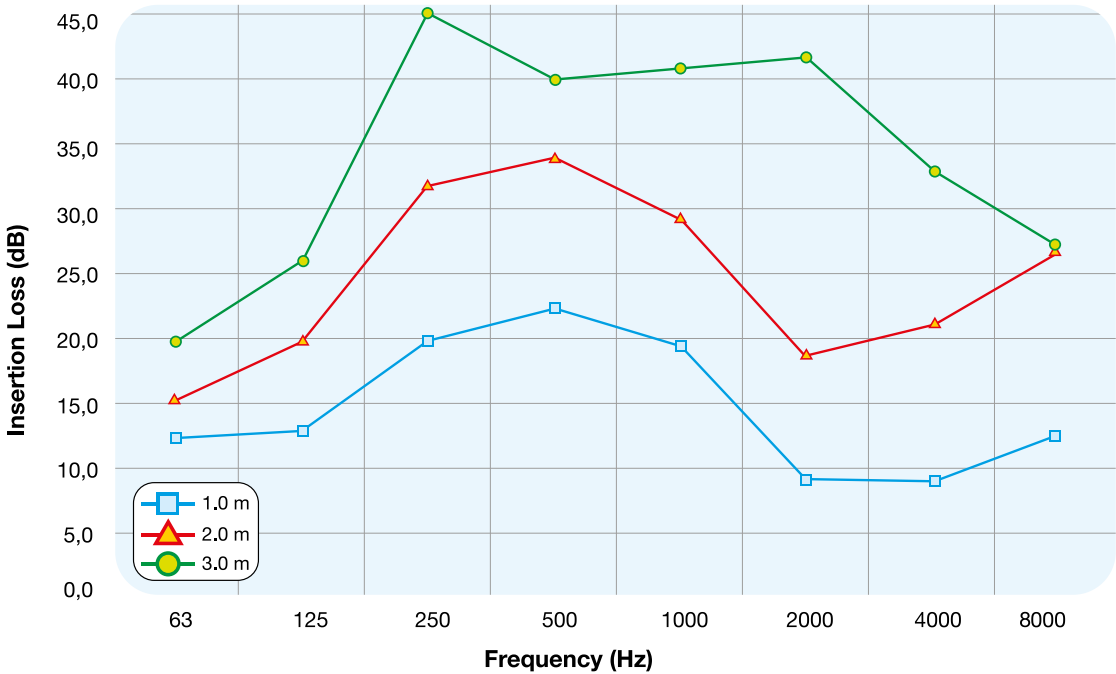
SONOAFS-ALU.F - Ø 102 mm
