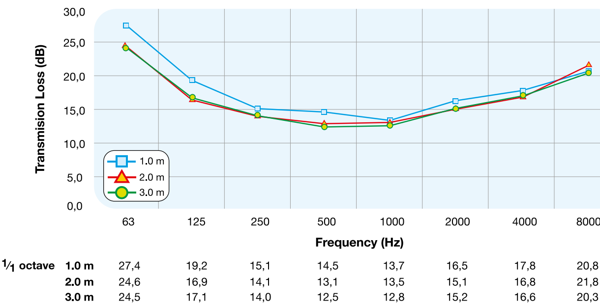
SONOAFS-ALU.F - Ø 203 mm
