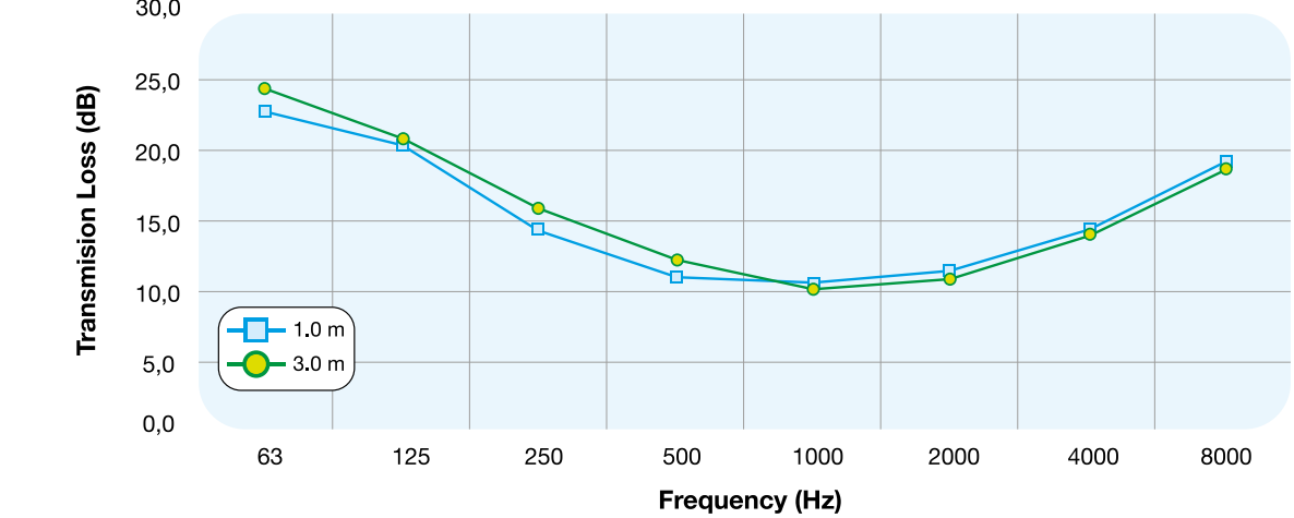
SONOAFS-NW.P - Ø 127 mm
