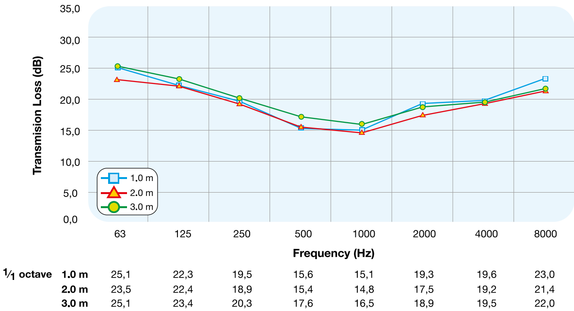
SONOAFS-ALU.F - Ø 127 mm
