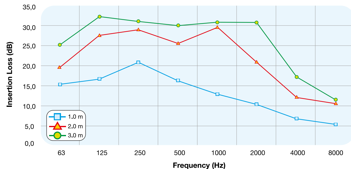
SONOAFS-ALU.F - Ø 254 mm
