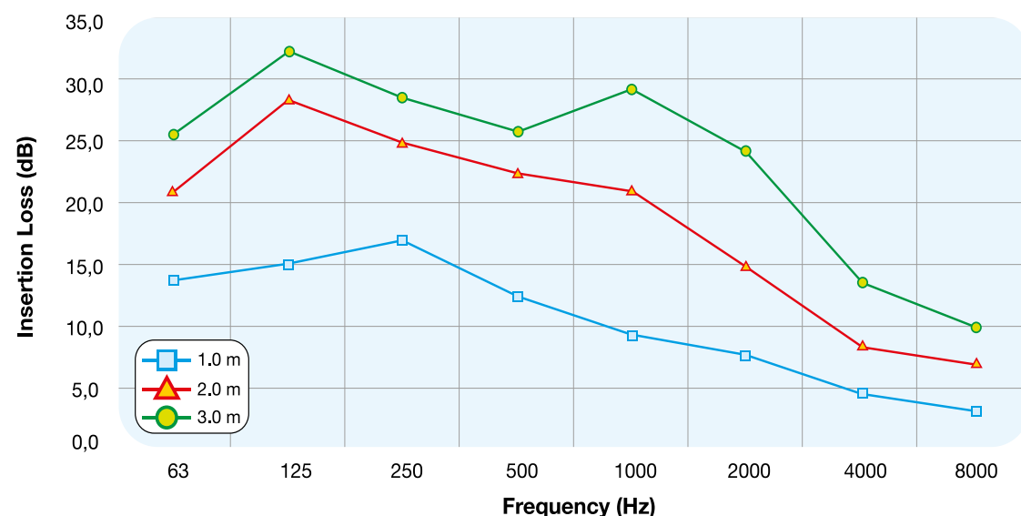
SONOAFS-ALU.F - Ø 315 mm
