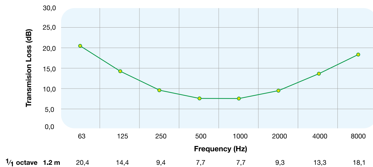
SOUNDROP AFS.P - Ø 200 mm - 0.6 m
