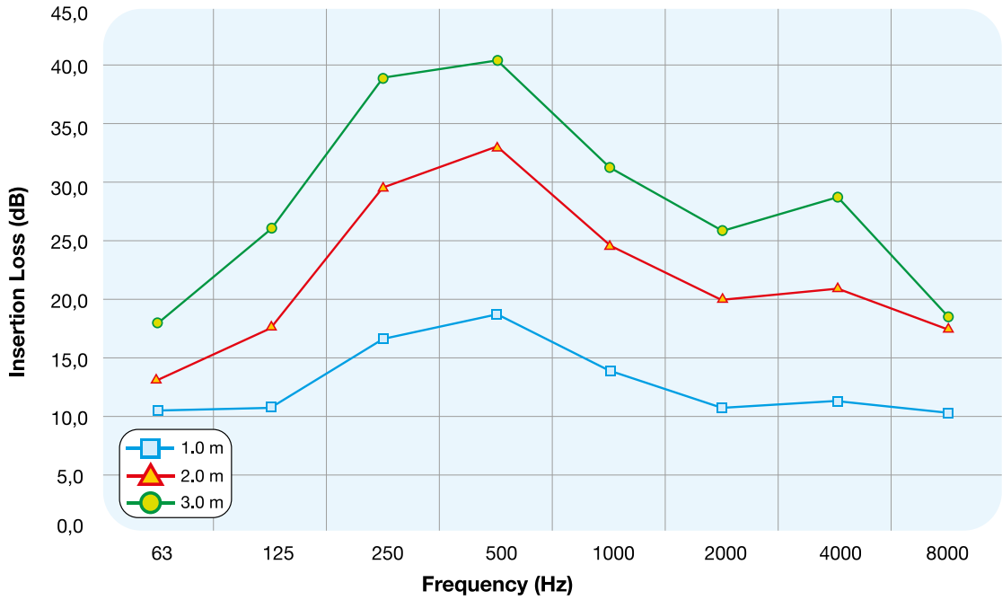
SONOAFS-ALU.F - Ø 127 mm
