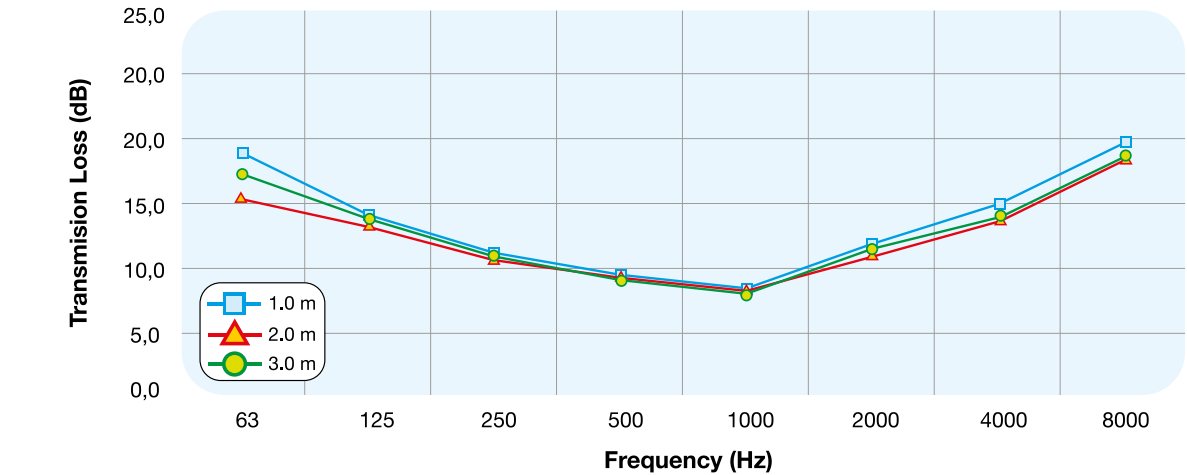
SONOAFS-ALU.F - Ø 254 mm
