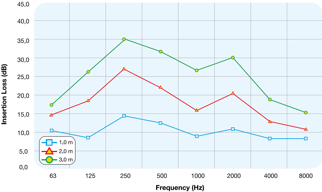
SONOAFS-ALU.F - Ø 203 mm
