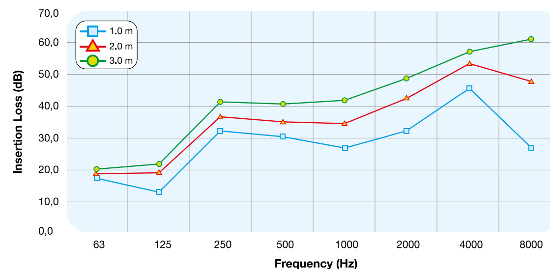
SONOAFS-NW.P - Ø 127 mm
